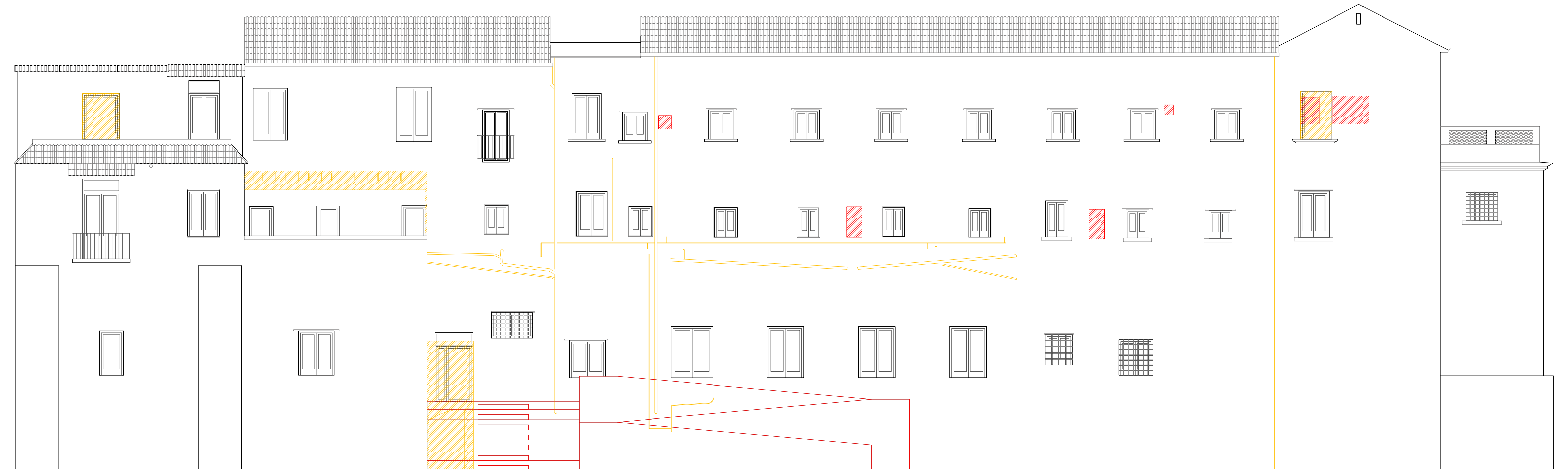
PROSPETTO O - SCALA 1:50
